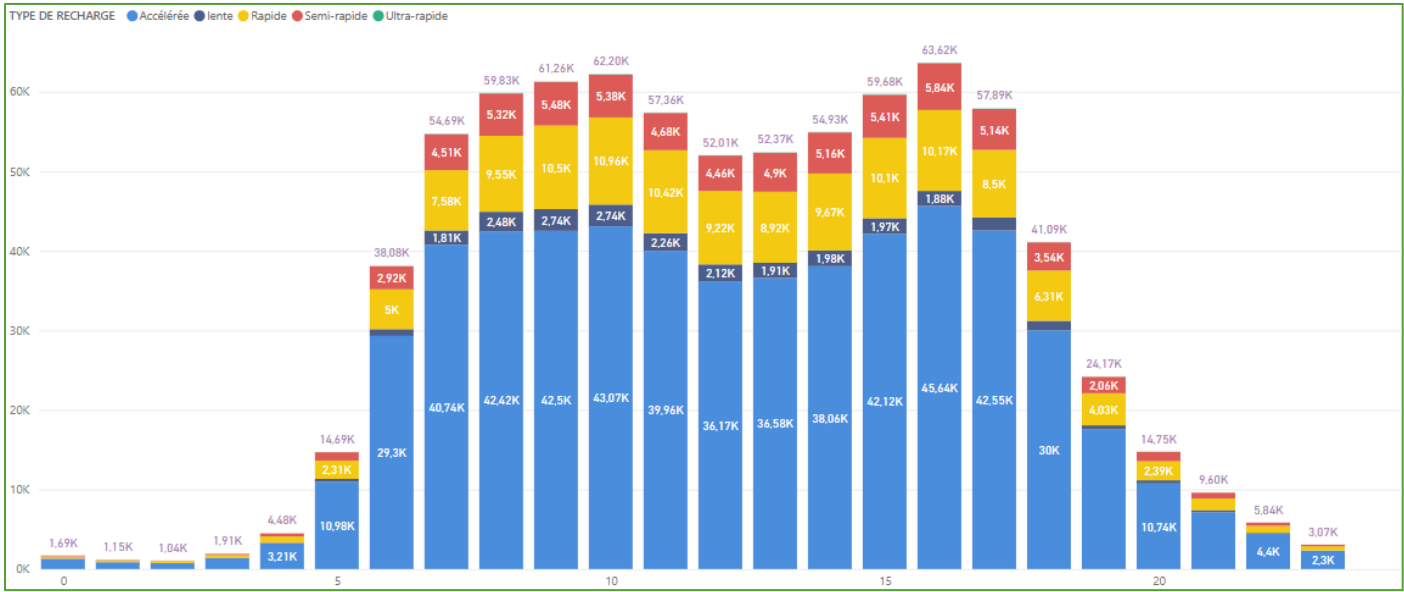
Répartition du nombre de sessions de charge en fonction de l'heure de lancement de la charge
