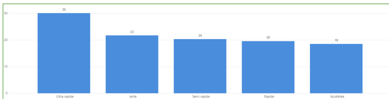
Consommation moyenne par sessions en kWh par de type de recharge
