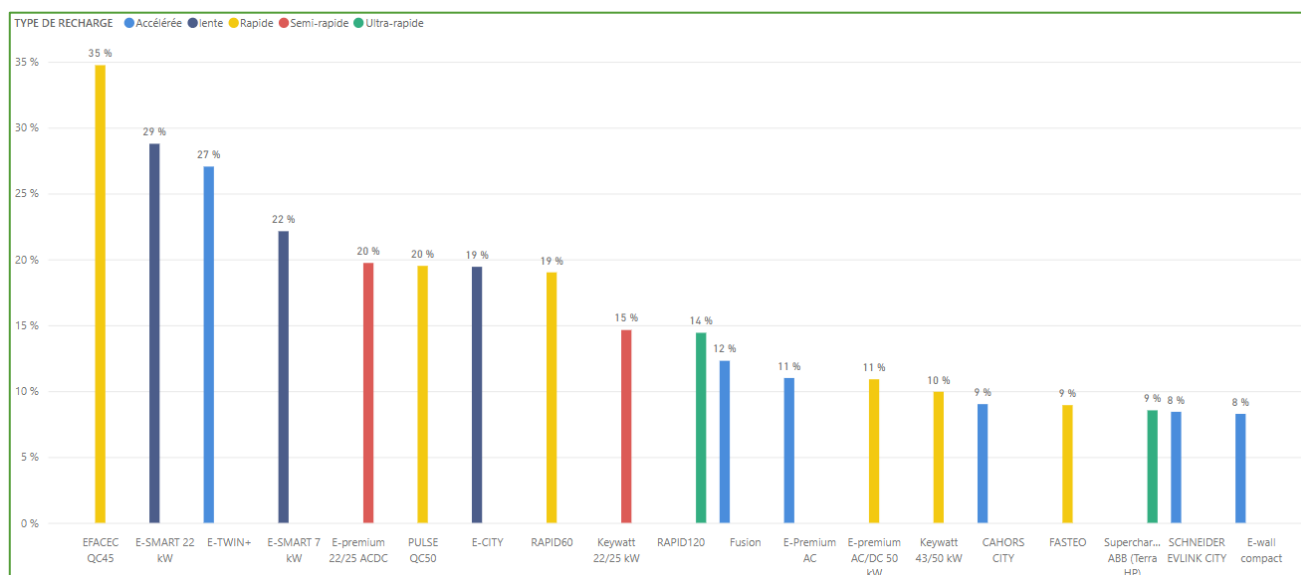
Taux de charge infructueuse par modèle de borne
