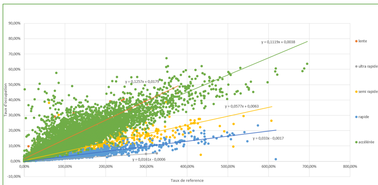
Corrélation entre le taux de référence et le taux d'occupation.
