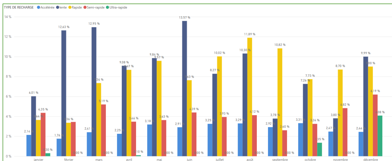
Moyenne du taux de perte de communication par mois et par type de borne
