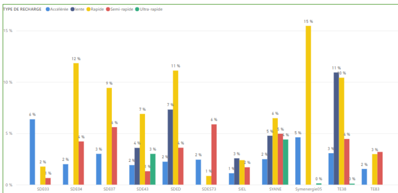
Moyenne du taux de perte de communication par syndicat et par type de borne
