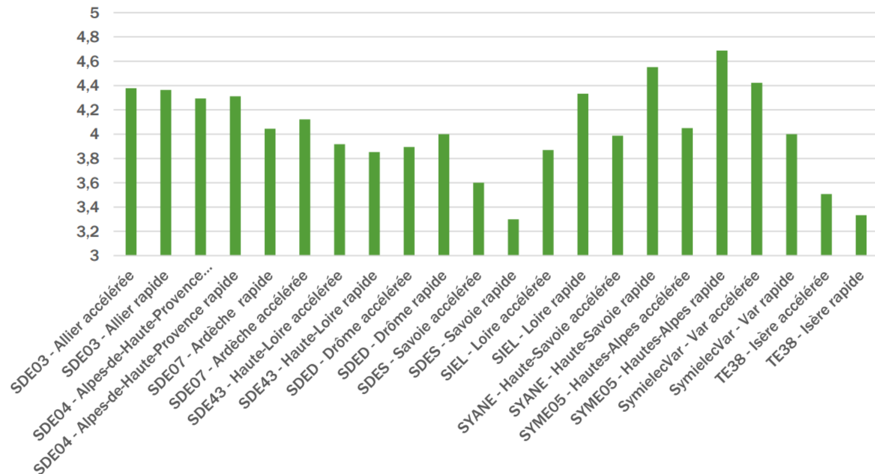
note moyenne par département et par type de borne
