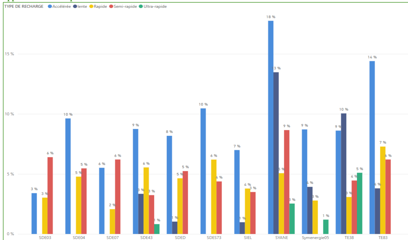
Moyenne du taux d'occupation annuelle par département et par type de borne
