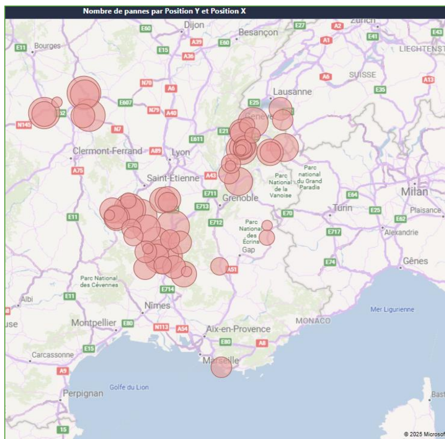
Localisation des bornes en fonction du nombre de pannes pour toutes les bornes en haut, et pour les bornes avec plus de 25 pannes dans l'année en bas
